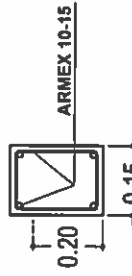
CADENA DE DESPLANTE Y NIVELACIÓN (CD-CN)
