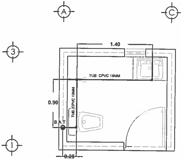
PLANTA INSTALACION HIDRAULICA
