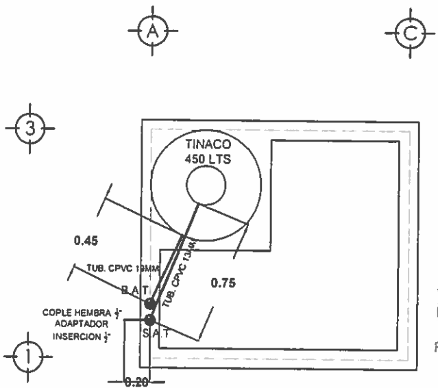
AZOTEA INSTALACION HIDRAULICA
