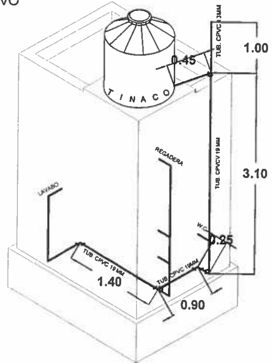
ISOMETRICO BAJANTE HIDRAULICO
