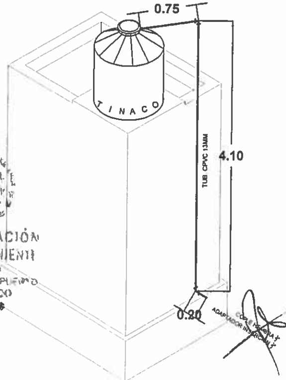
ISOMETRICO ALIMENTACION HIDRAULICA
