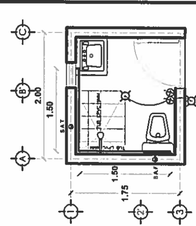
INSTALACION HIDRAULICA Y ELECTRICA
